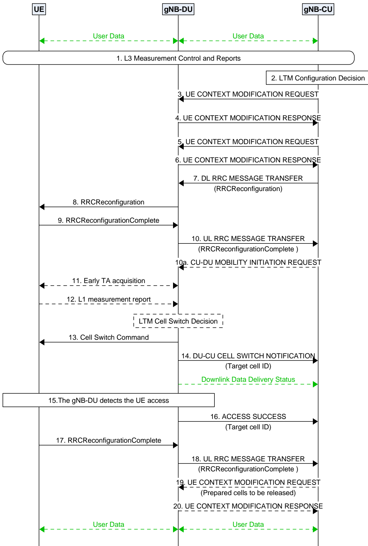
Figure 8.2.1.4-1: Intra-gNB-DU LTM
