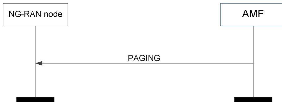
Figure 8.5.1.2-1: Paging
