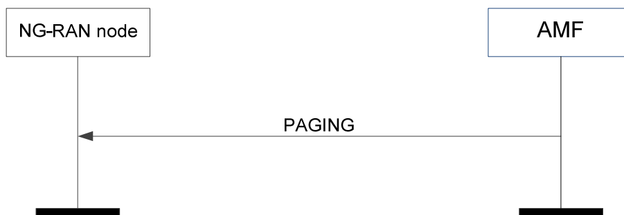
Figure 8.5.1.2-1: Paging
