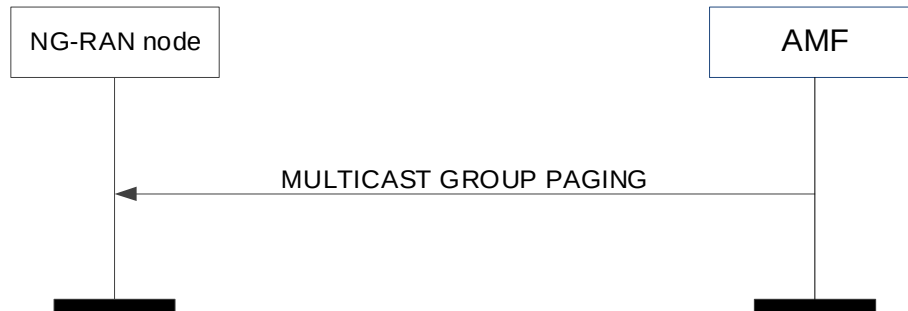
Figure 8.5.2.2-1: Multicast Group Paging
